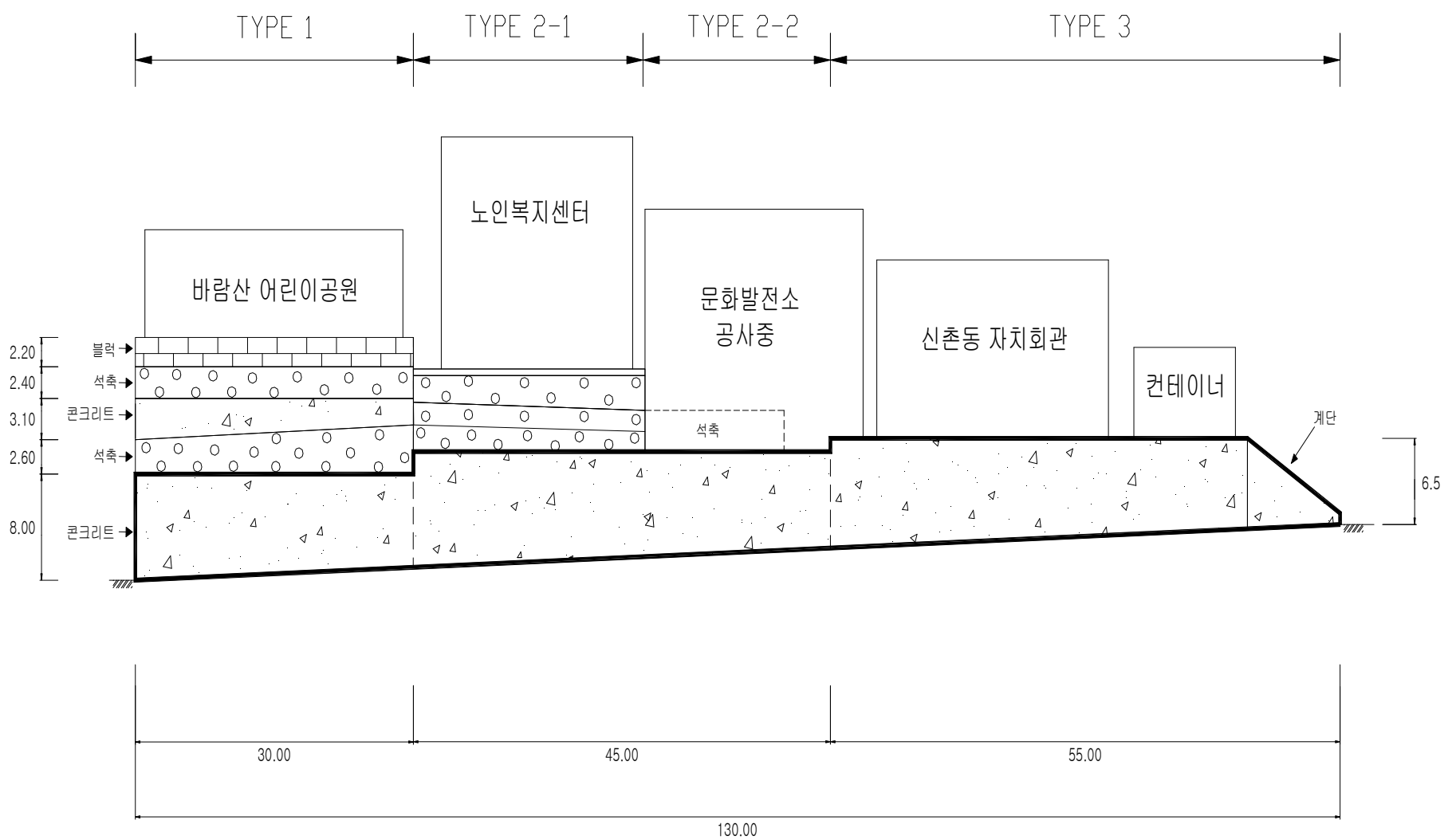
정면도(복원도면)
